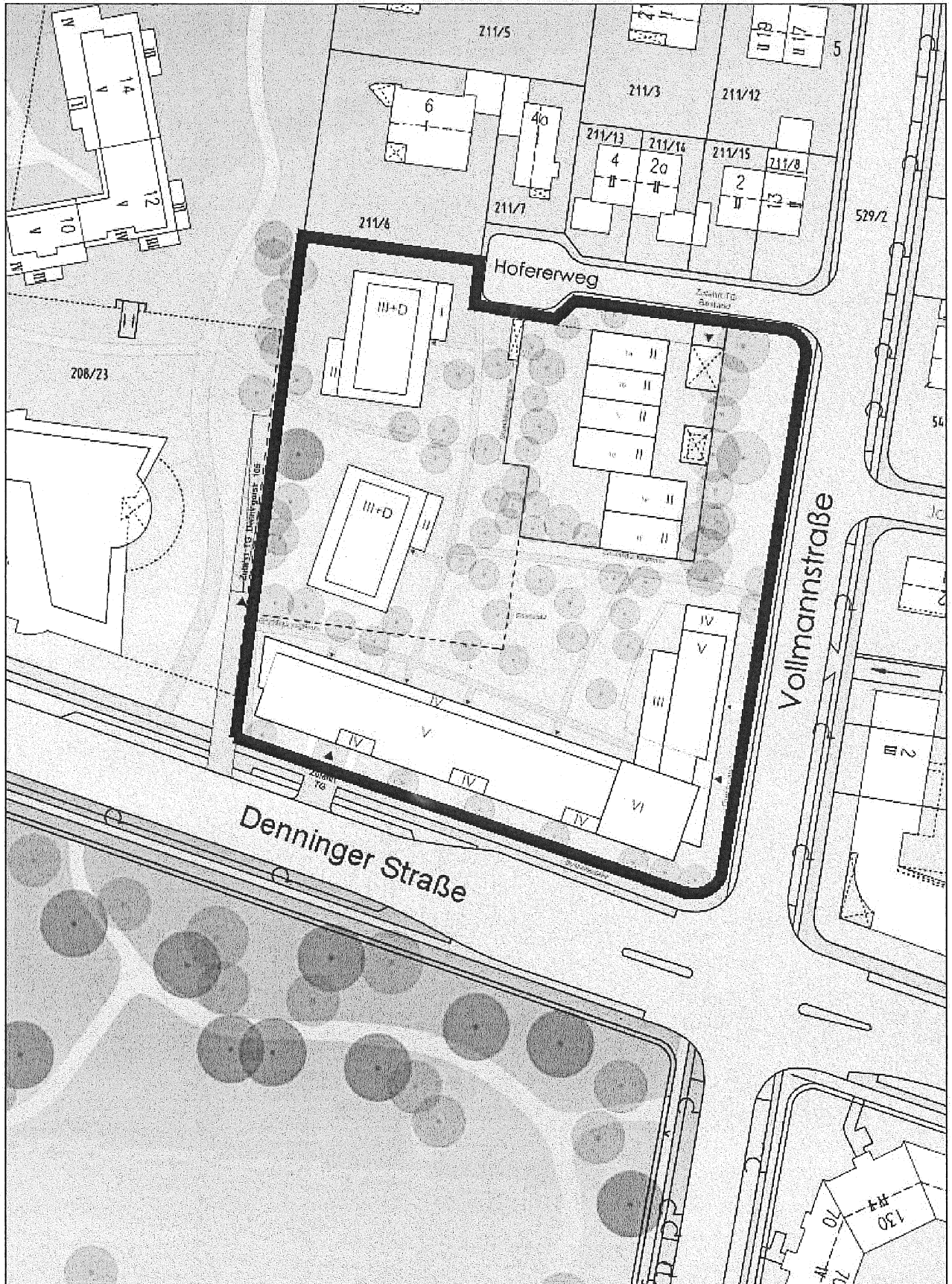
PLANUNGSKONZEPT
