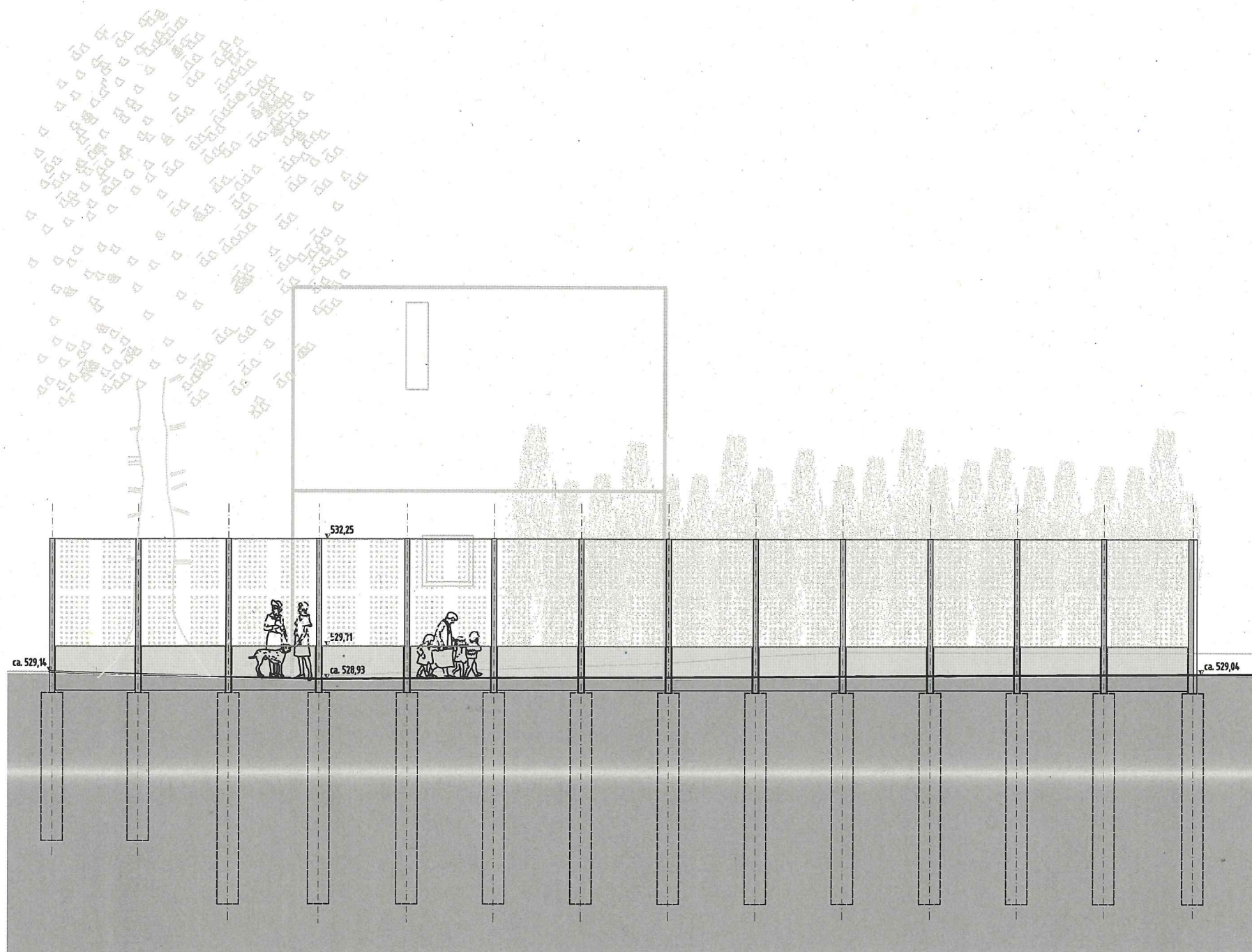
Ansicht West (abgewickelt)
