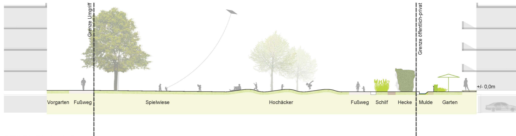
SCHNITT "Hochäcker" Maßstab 1:250
