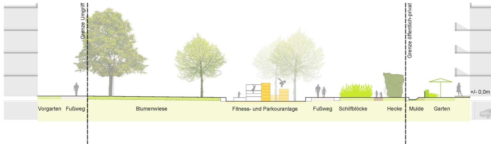
SCHNITT "Kistenstapel" Maßstab 1:250
