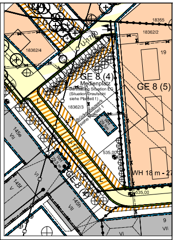
Planteil 2: Situation EG Ausschnitt Brückenbauwerk (Situation Draufsicht in Planteil 1) M 1:500
