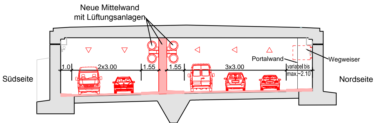
Schnitt A - A
