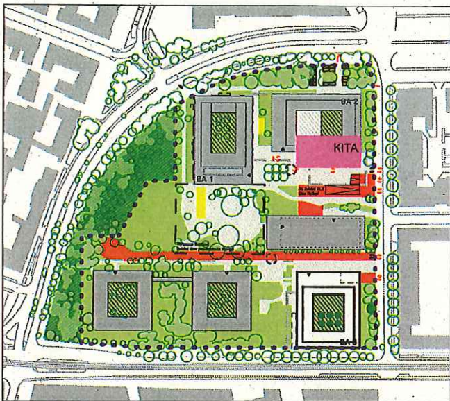
Bauabschnitt 3
