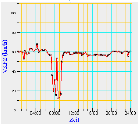
Anlage 1: Geschwindigkeitstageswerte an verschiedenen Detektoren – Richtung Ost → West
