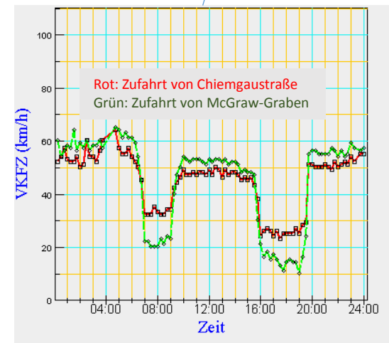
Anlage 1: Geschwindigkeitstageswerte an verschiedenen Detektoren – Richtung Ost → West
