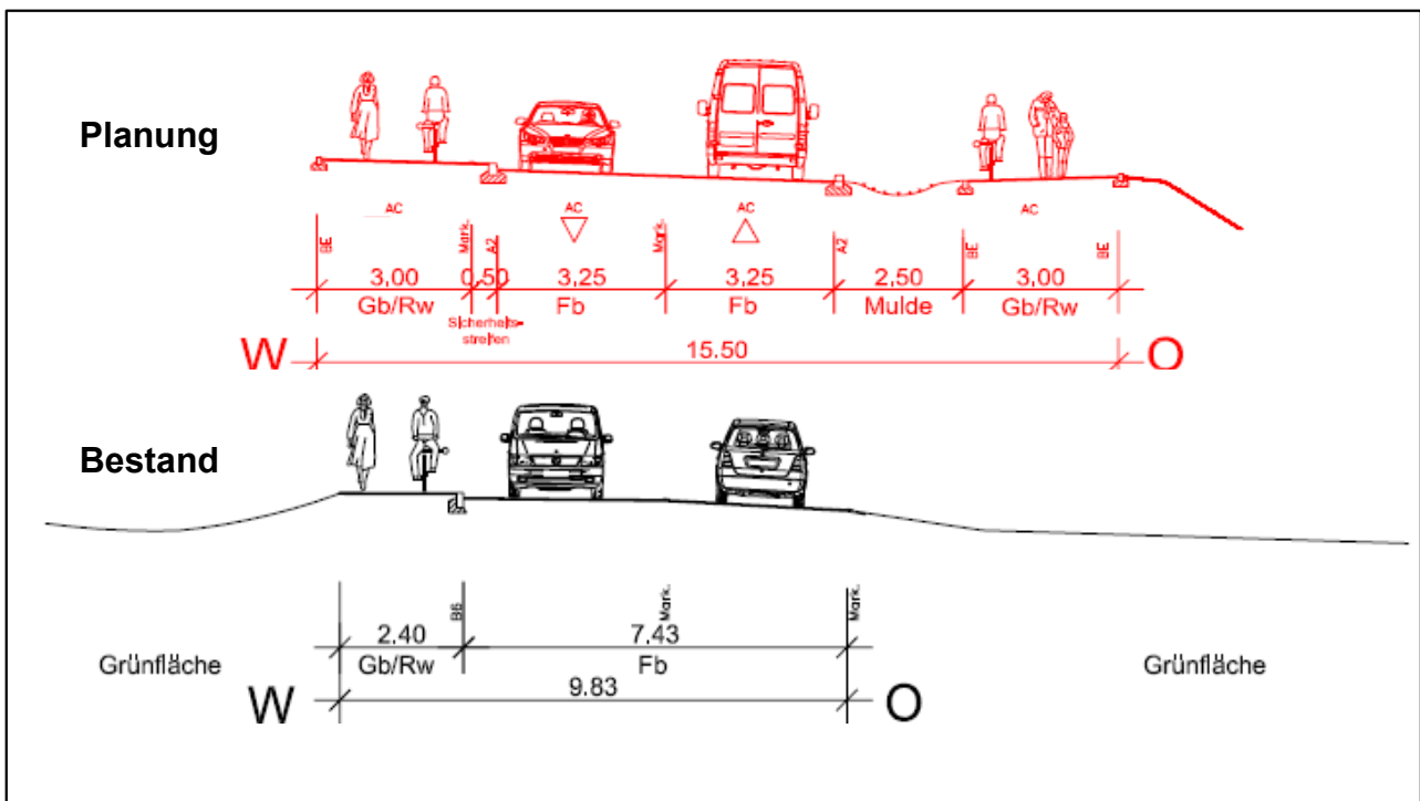
Querschnitt 2, Regelquerschnitt zwischen der Noestraße und der Siemensallee
