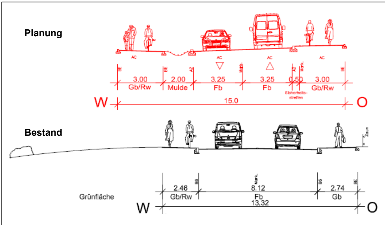
Querschnitt 1, Regelquerschnitt zwischen der Ascholdingner Straße und der Beuerberger Straße
