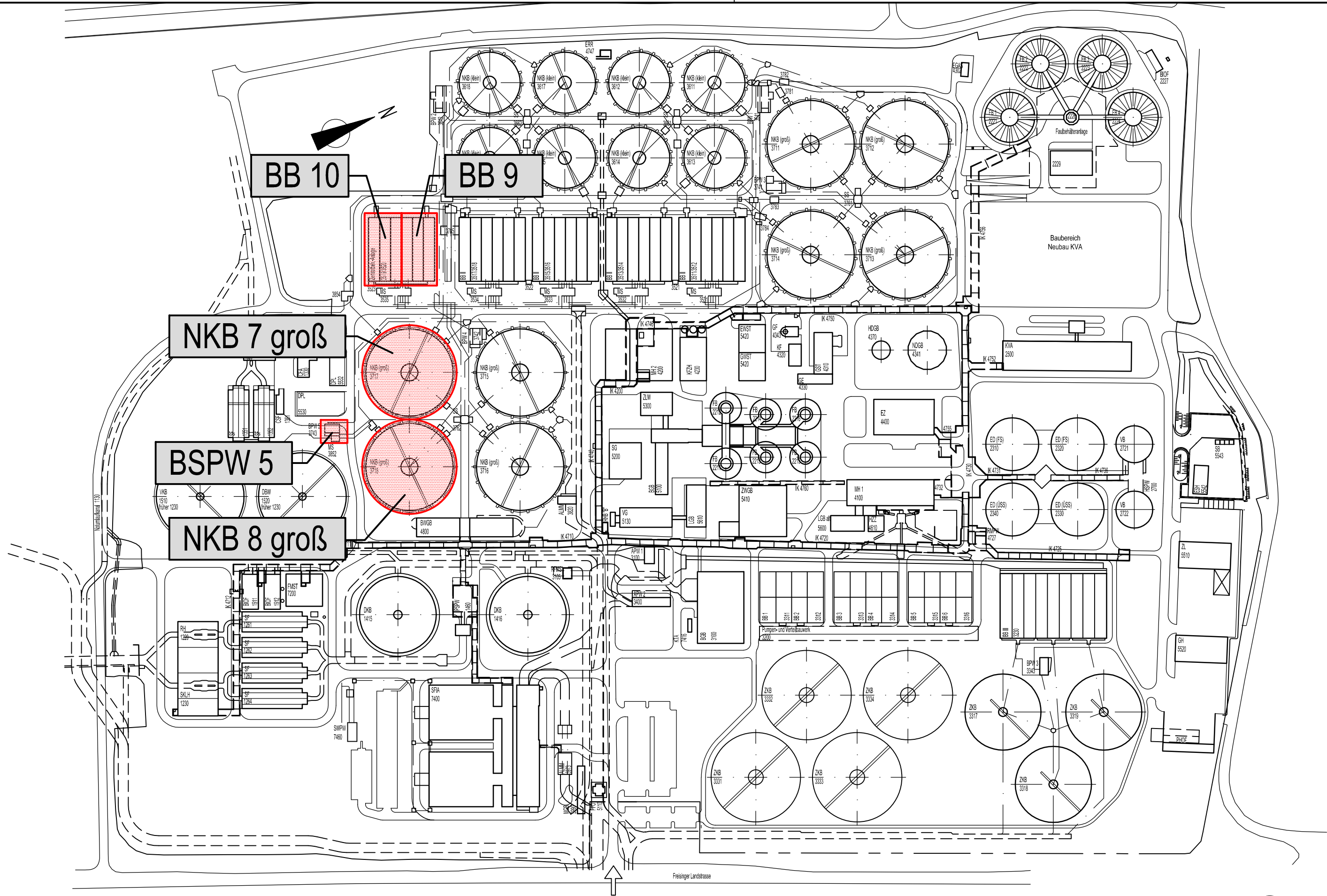
Anlage C Übersichtslageplan
