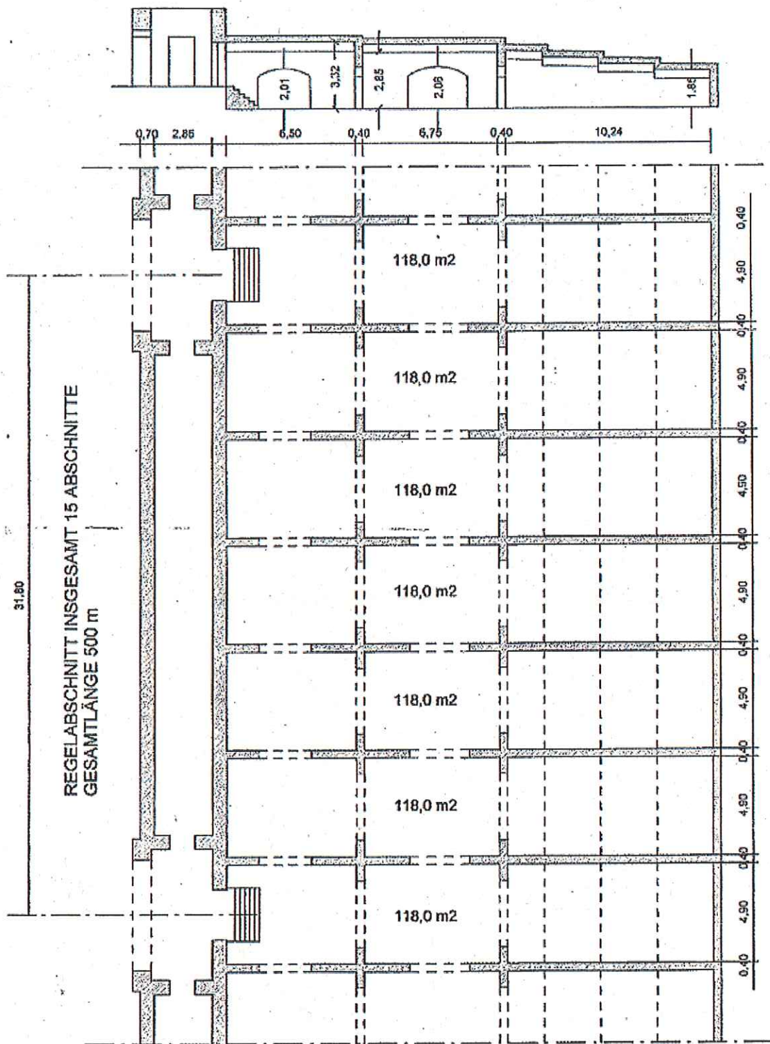
Bild 5: Grundriss und Schnitt eines Regelabschnittes der Tribüne, Länge ca. 32 m, Breite ca. 27 m, lichte Höhe ca. 3,3 m bis ca. 1,8 m
