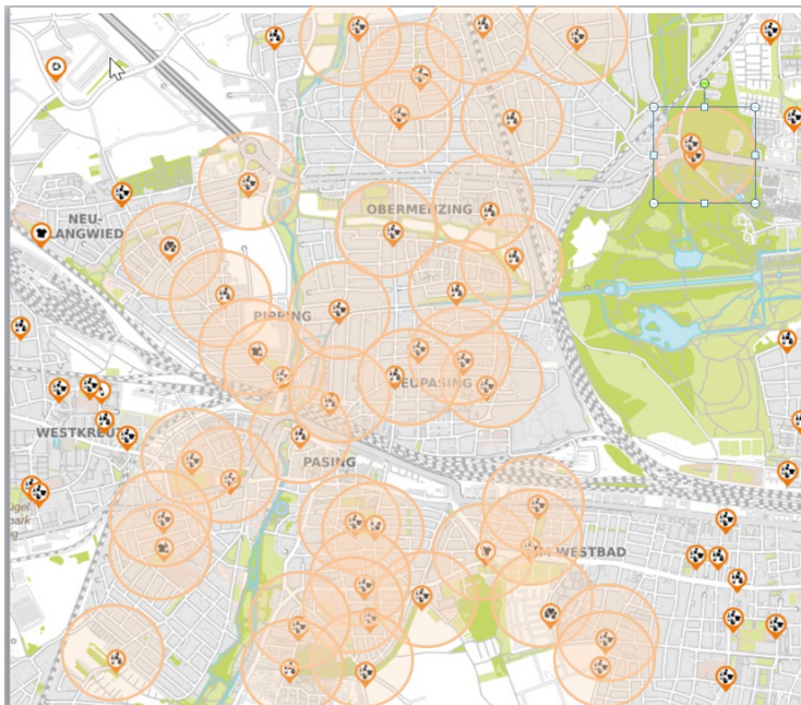
Standorte der Wertstoffsammelinseln im BA 21 mit 300 m Radius nach https://geoportal.muenchen.de/portal/awm
