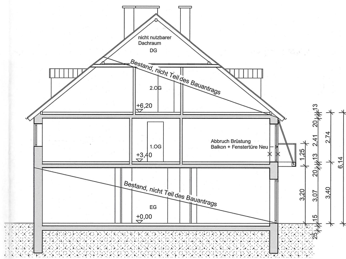
Schnitt B-B
