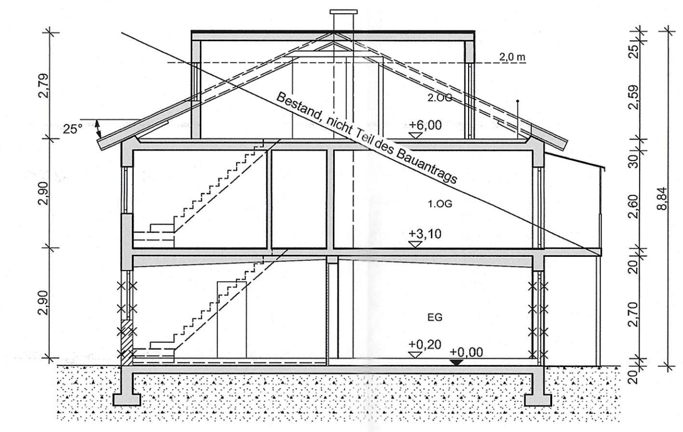
Schnitt A-A
