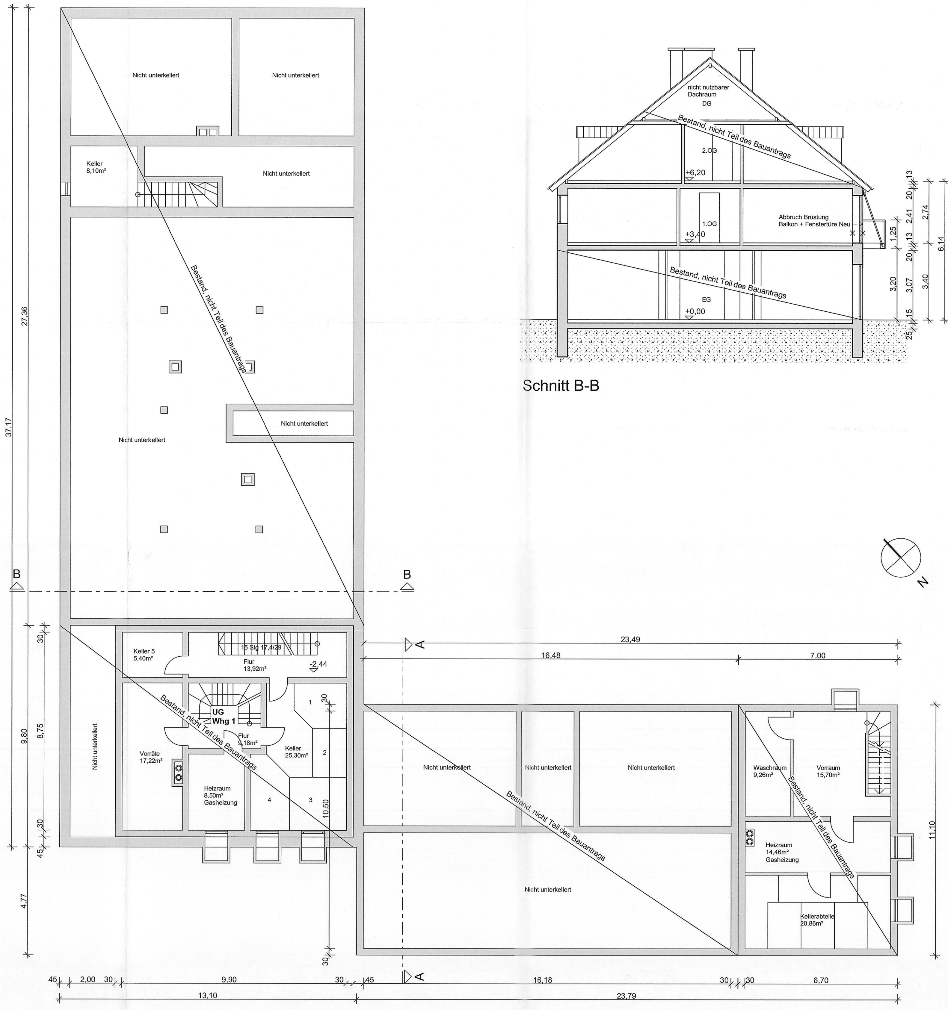
Grundriss UG
