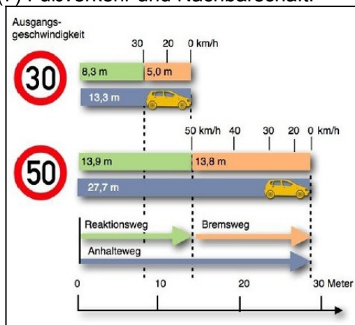
Anhalteweg bei Tempo 30 v. Tempo 50 bei einer Reaktionszeit von einer Sekunde und einer Bremsverzögerung von 6,5 \text{ m/s}^2 (entspricht trockener Fahrbahn, bei Nässe länger) (Grafik: Hubert Ströhle für ADFC)
