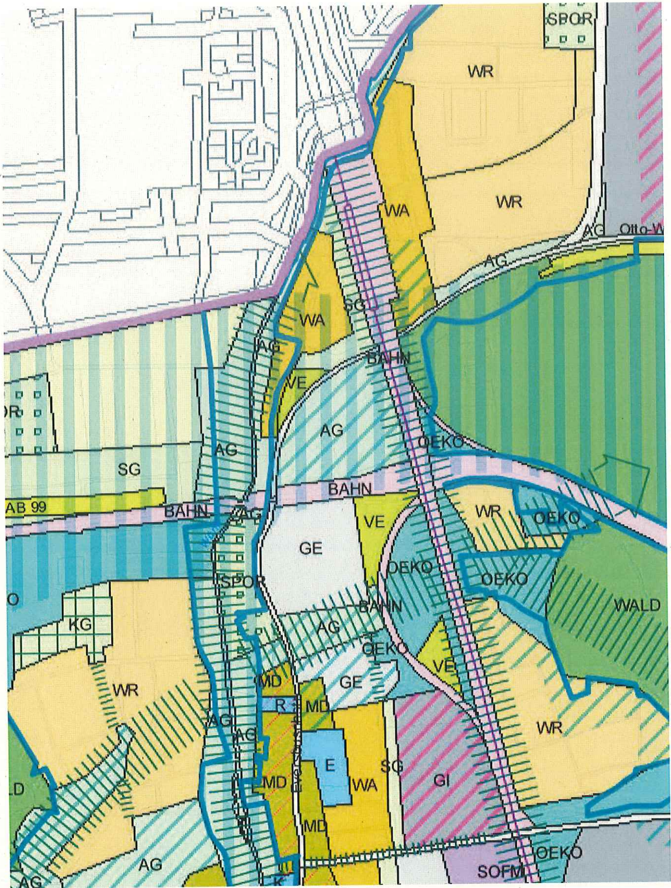
Bebauungsplan Eversbuschstraße "Hirmerei" Ausschnitt Flächennutzungsplan
