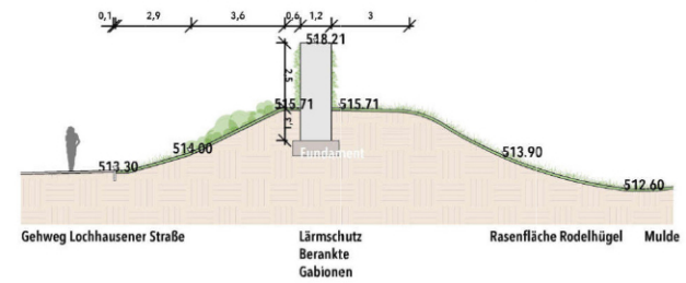
Schnitt E-E' M 1:200
