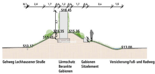
Schnitt F-F' M 1:200
