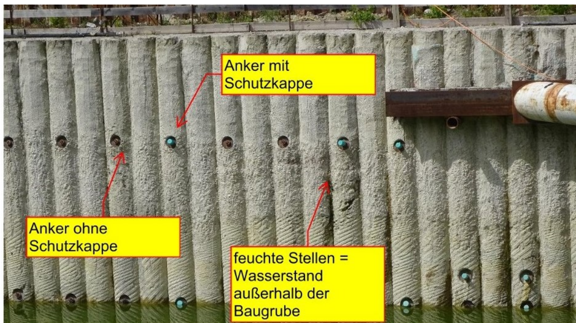
Abbildung 1: Ausschnitt Ansicht nördliche Baugrubenwand
